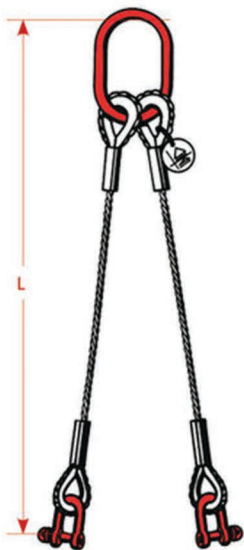
1216. Élingue câble
