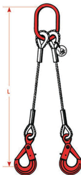
1217. Élingue câble
