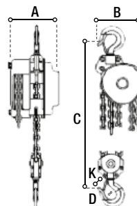
Capacité 20 t
