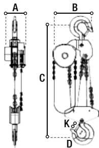
Capacité 10 t
